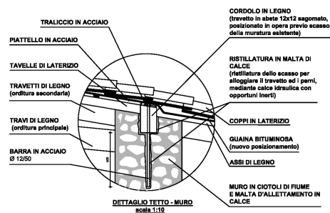
Progetto del cordolo
